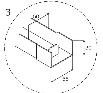
Onderrail
